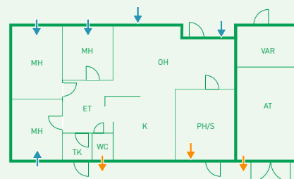
Fresh TL98F Korvausilmaventtiili 5 kpl asennettuna*
